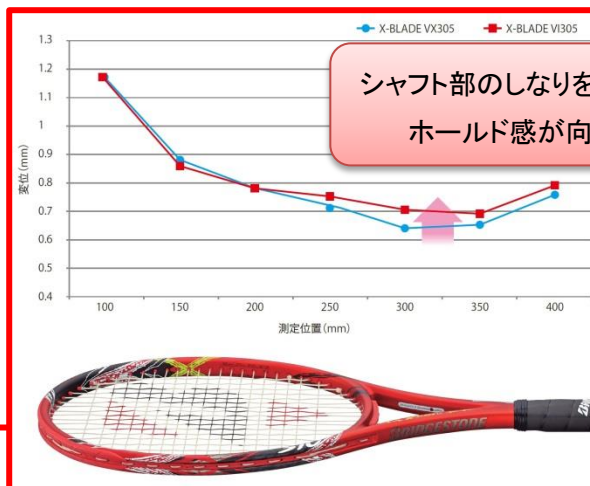
薄型ボックス形状剛性分布
