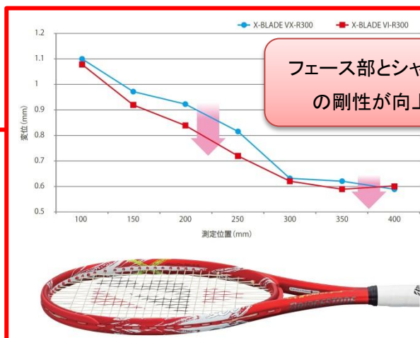
中厚ラウンド形状剛性分布
